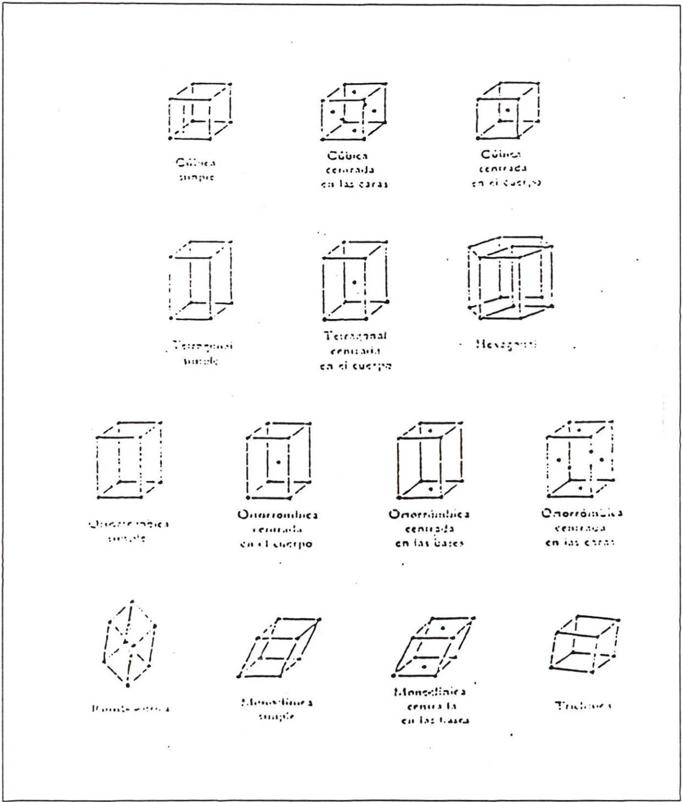
Los siete sistemas de estructura cristalina y las 14 redes de Bravais
