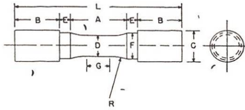
DIMENSIONS
