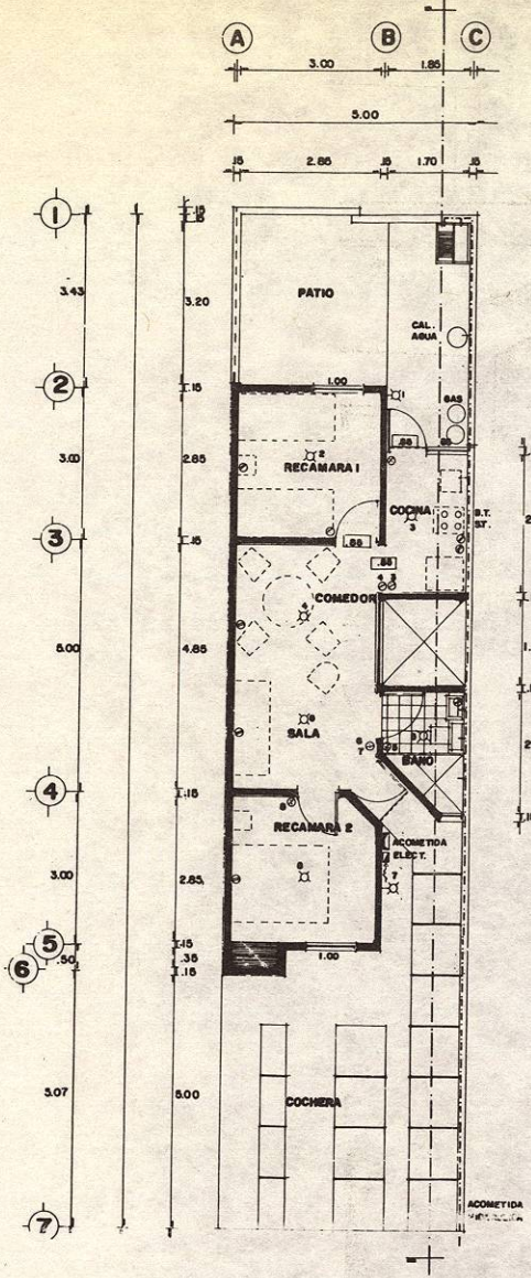
planta arquitectonica
