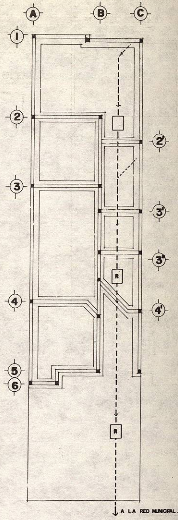
planta cimentacion
