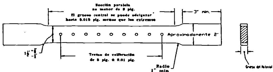
(c) Probeta rectangular estándar con tramo de calibración de 8 plg. para ensaye de metales en forma de placa, lámina, etc., con grueso de 3/16 plg. o más.
