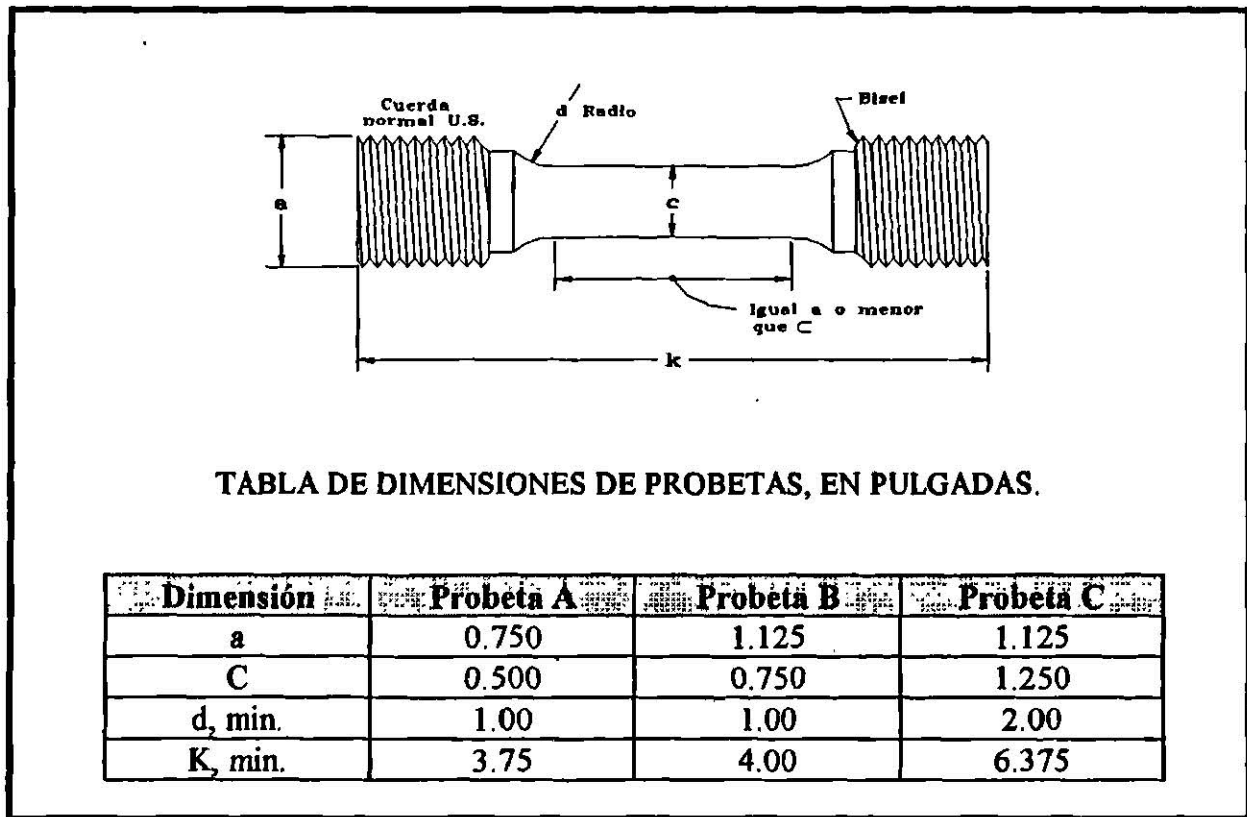
Figura 3.11 Estándar para Hierro fundido A.S.T.M. E-8, A 48
