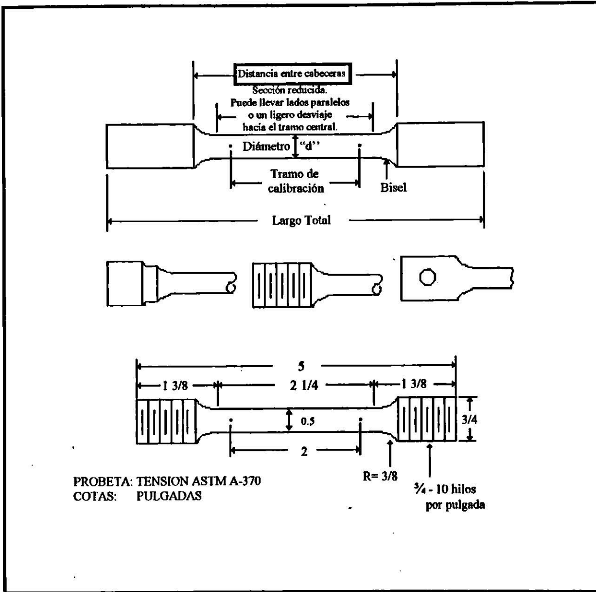
Figura 3.7 Tipos de extremos para probetas de tensión
