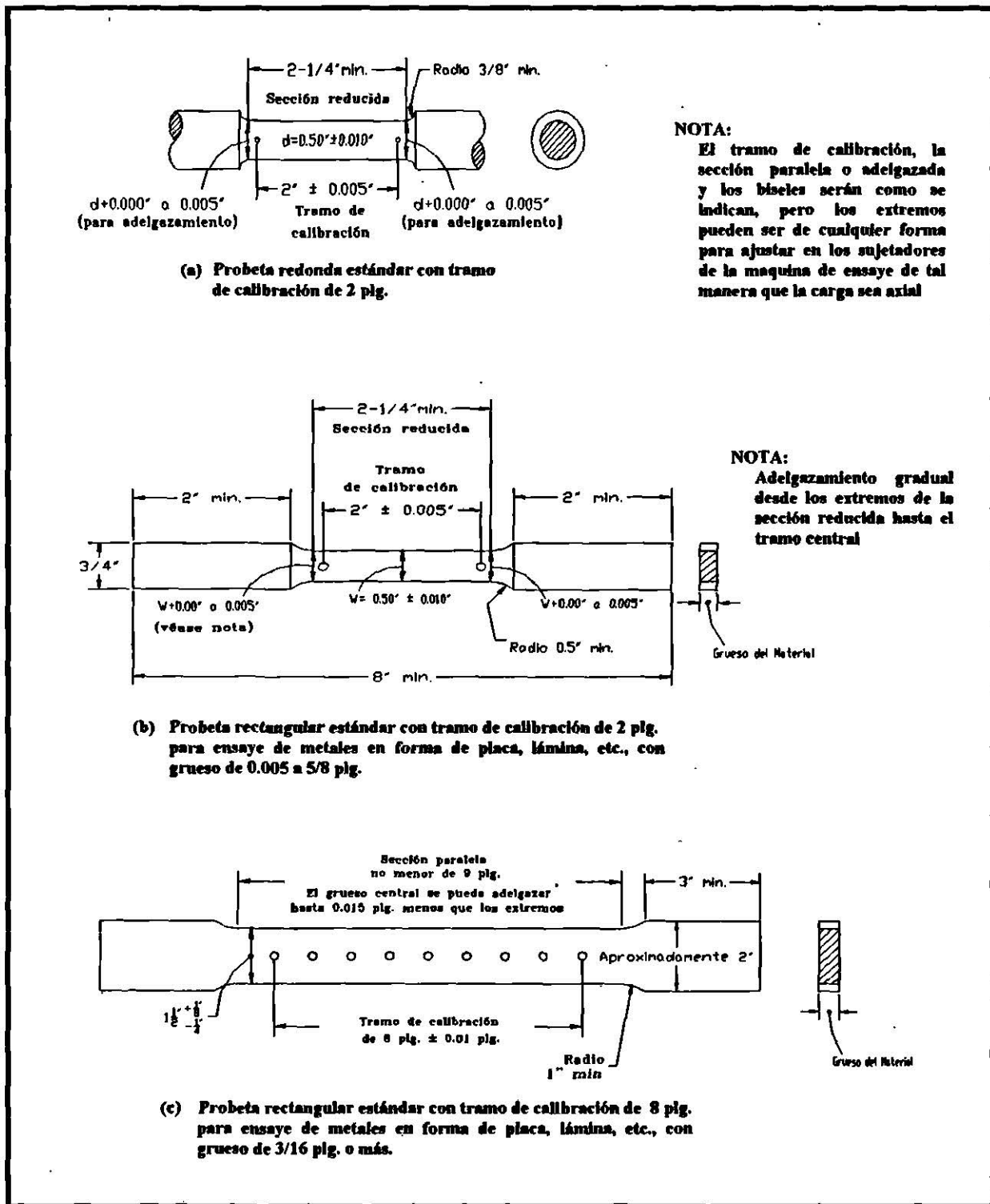
Figura 3.10 Estándar A.S.T.M. E-8, A 370 para ensayos estáticos de tensión en metales dúctiles
