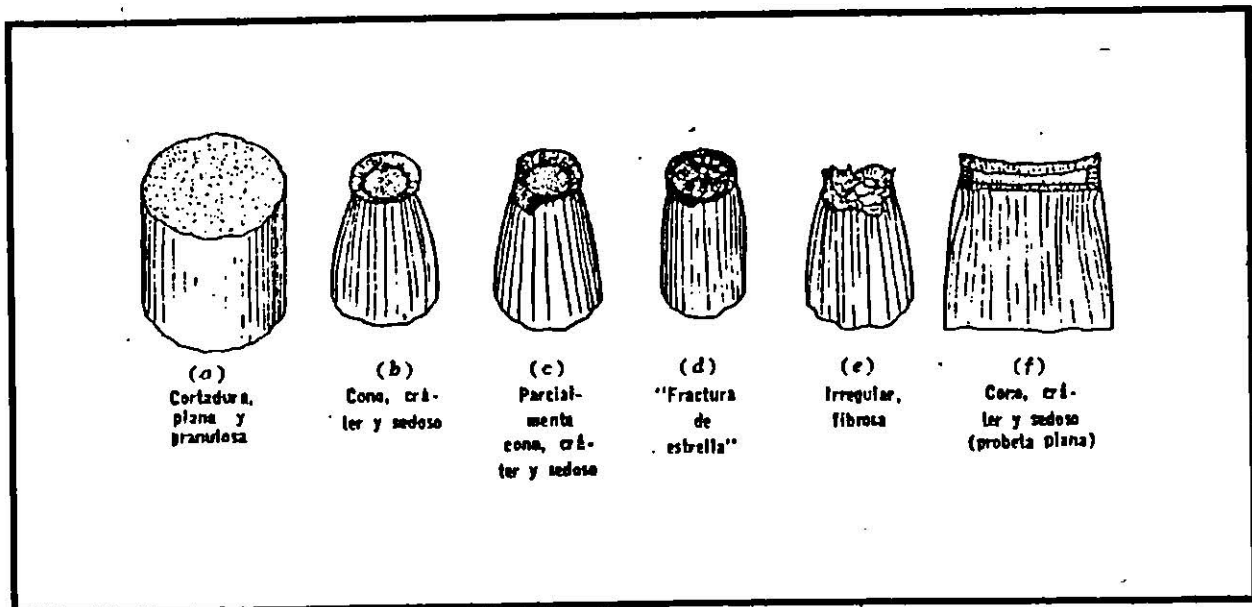
Figura 3.13 Fracturas típicas por tensión en metales.
