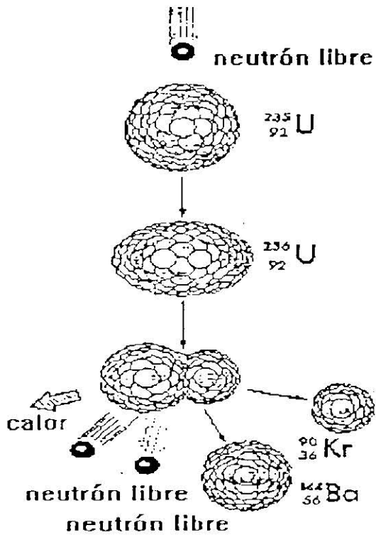
REACCION DE FISION
