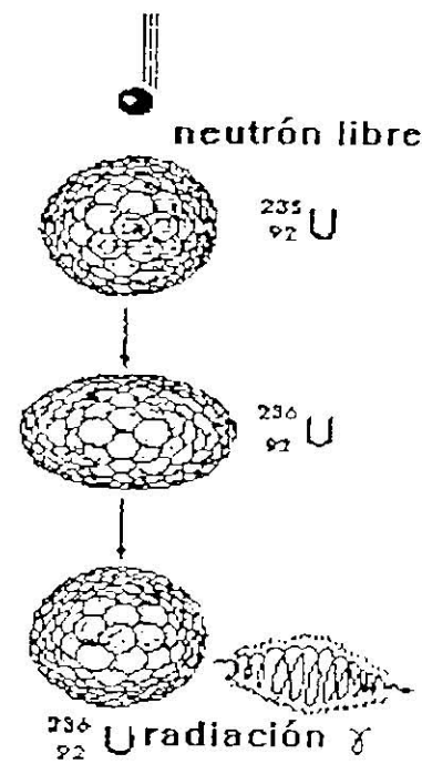
REACCION DE CAPTURA
