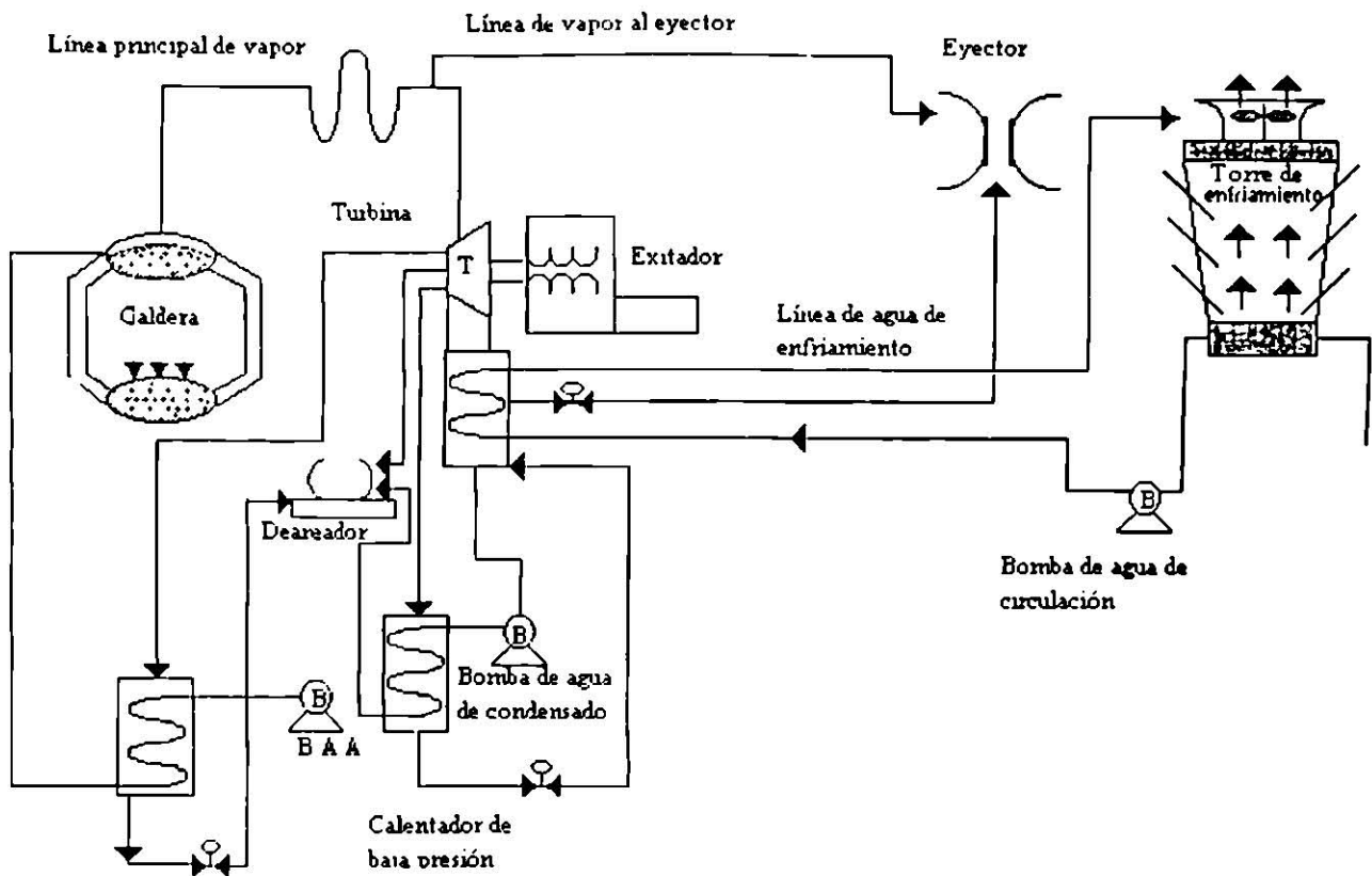
Fig. 2.1 Ciclo de agua-vapor de una central termoelectrica.
