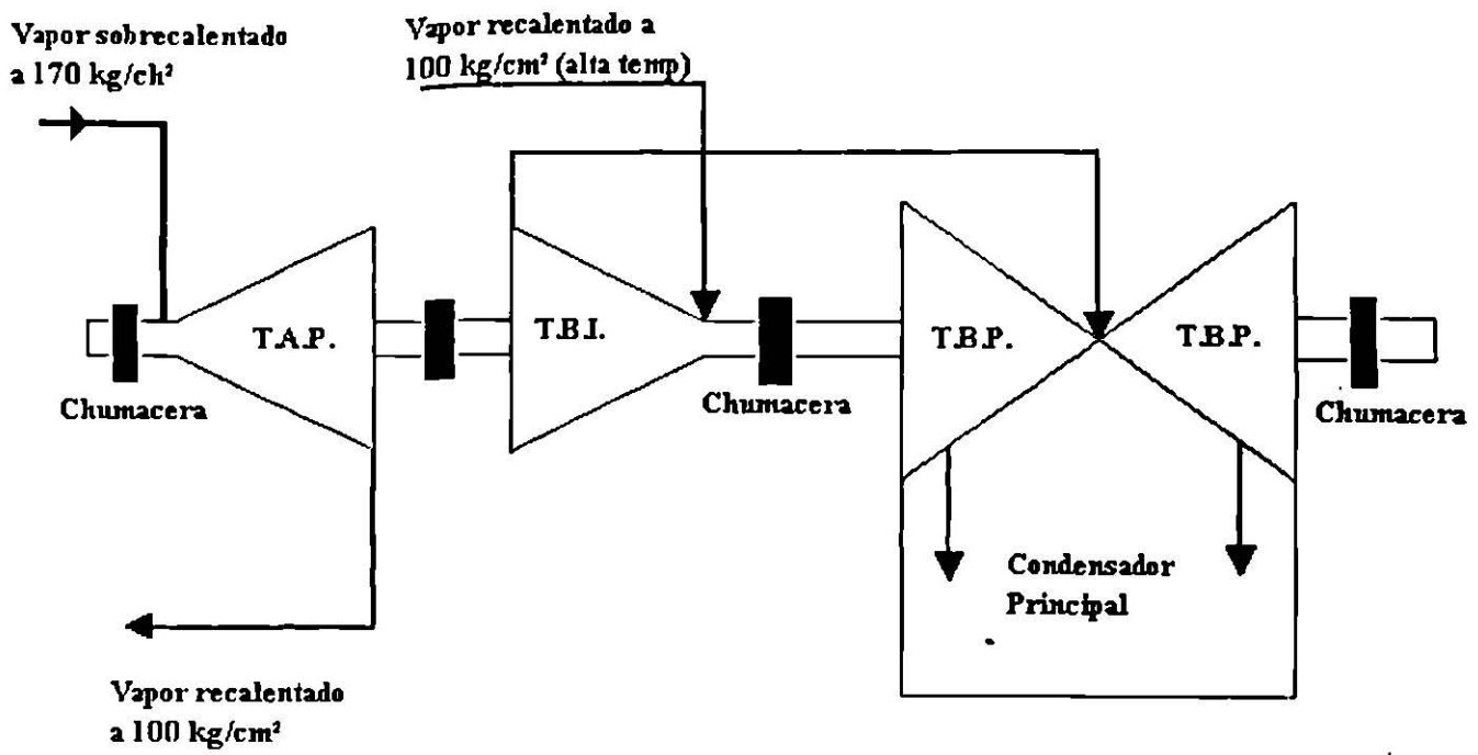
Fig. 4.1 Arreglo de Turbinas de Gran Capacidad.
