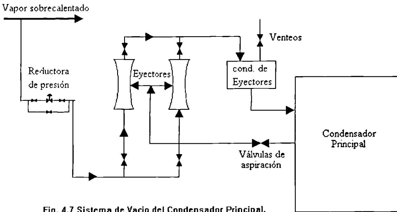
Fig. 4.7 Sistema de Vacío del Condensador Principal.
