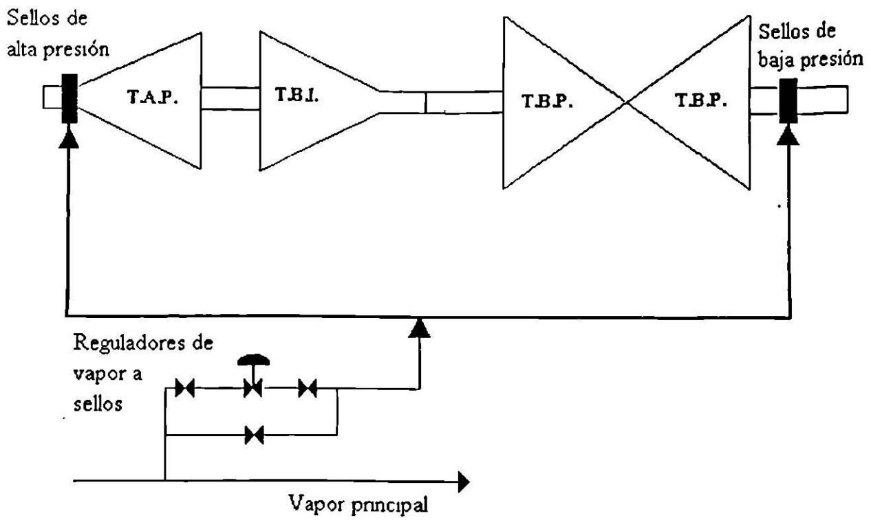
Fig. 4.5 Arreglo de Vapor a Sellos.
