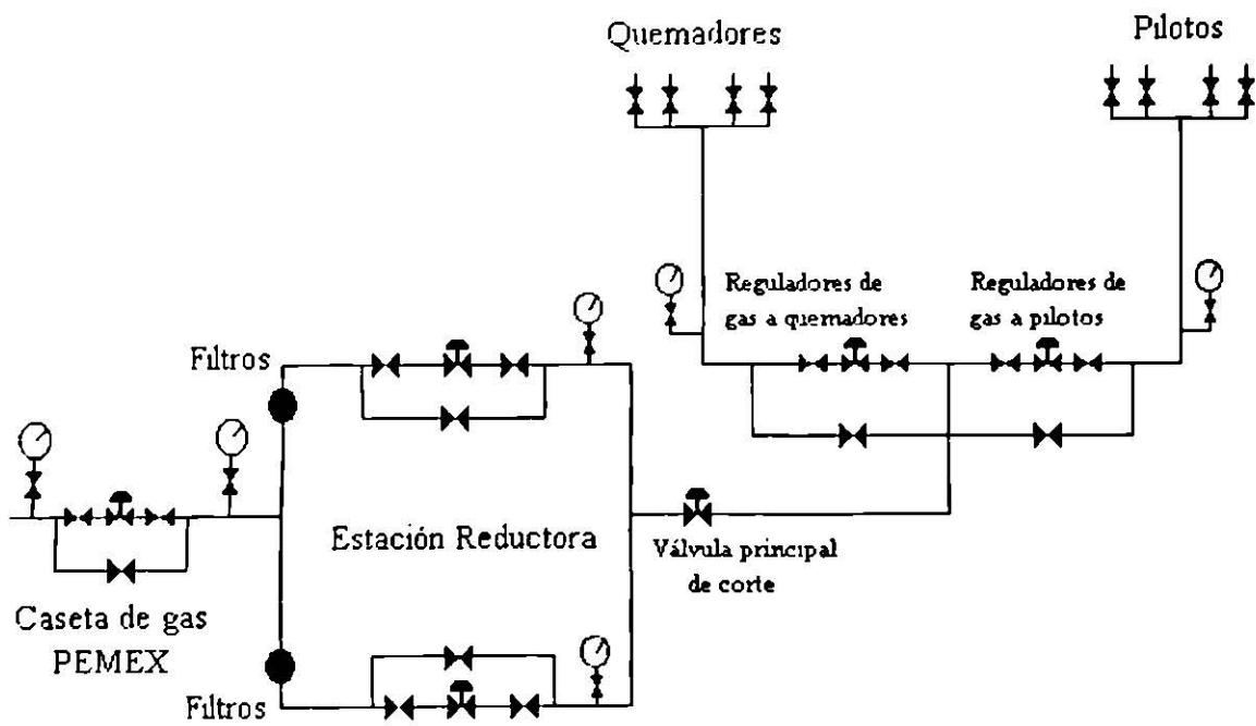
Fig. 3.2 Sistema de Suministro de Gas Natural a una Central Termoelectrica.
