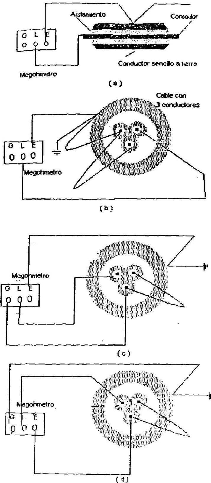
Figura 2.4 Conexiones de la prueba de cable para medición de la resistencia de aislamiento: (a) Conexión para la prueba de un conductor sencillo y un conductor a tierra. (b) Conexión para un cable de tres conductores, un conductor a otro conductor y el envoltorio a tierra. (c) Conexión para un cable de tres conductores, un conductor a la vaina y a tierra y dos conductores protegidos. (d) Conexión para un cable de tres, un conductor a todos los otros conductores sin pérdidas por tierra.
