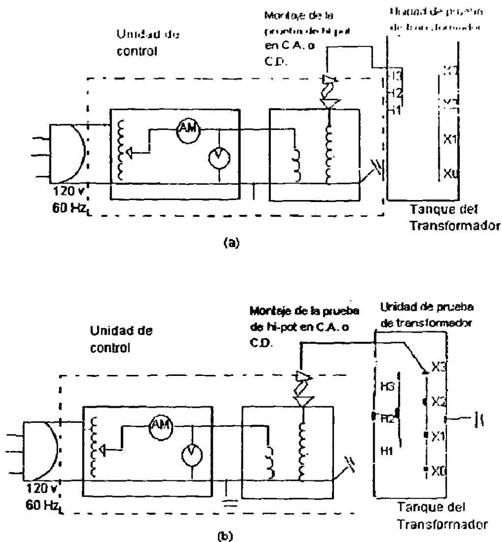
Figura 2.3 Conexión de la prueba de alto voltaje del transformador (HI-POT) a: Conexión de la prueba HI-POT en las bobinas de alta. (b) Conexión de la prueba de HI-POT en las bobinas de baja.
