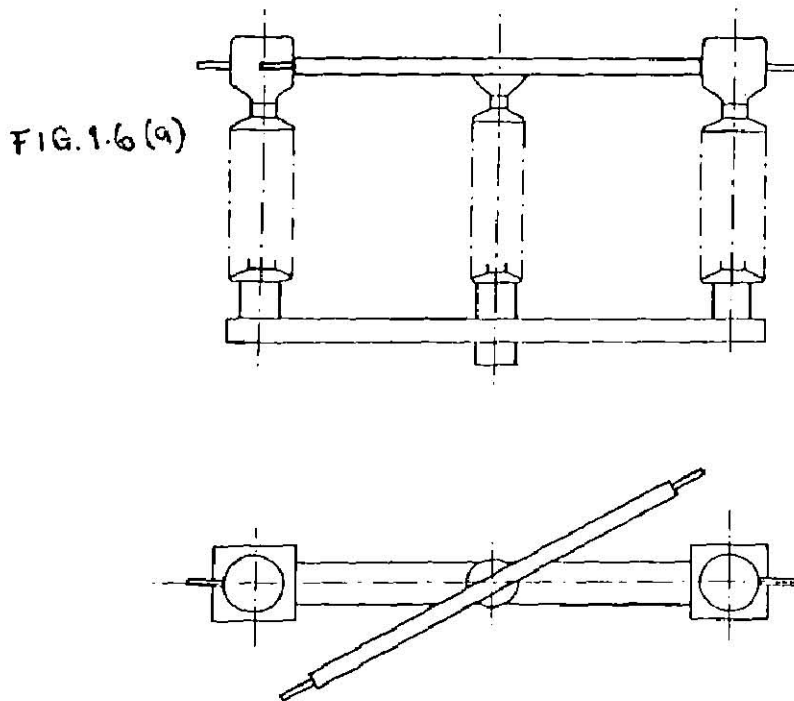
CUCHILLA DESCONECTADORA DE TRES COLUMNAS CON ACCIONAMIENTO EN LA COLUMNA CENTRAL.
