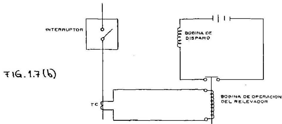
La representación típica del circuito de un relevador
