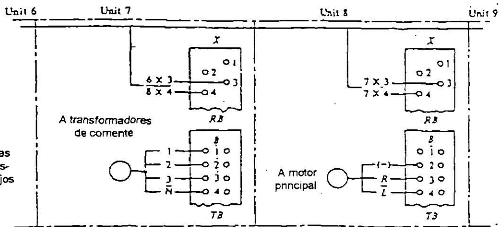
(c) Diagrama de interconexion
