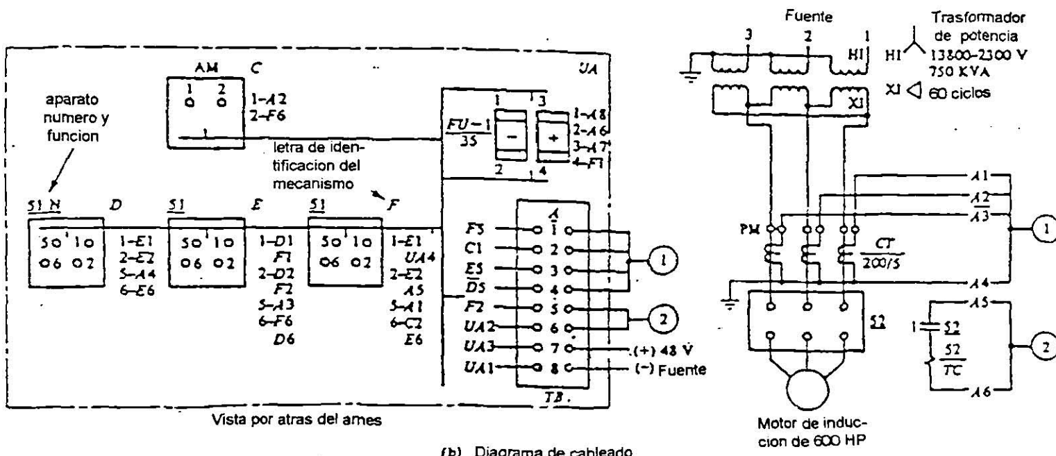
(b) Diagrama de cableado
