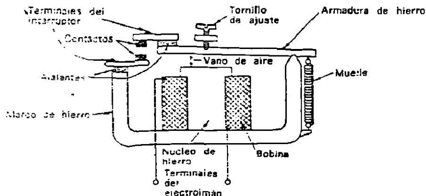
FIG. 1.7 (a) Relé banco.
