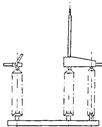
CUCHILLA DESCONECTADORA DE TRES COLUMNAS CON ACCIONAMIENTO EN LA COLUMNA CENTRAL.
