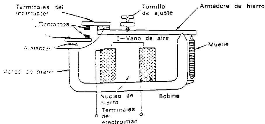
FIG 1.3(a) Relé básico
