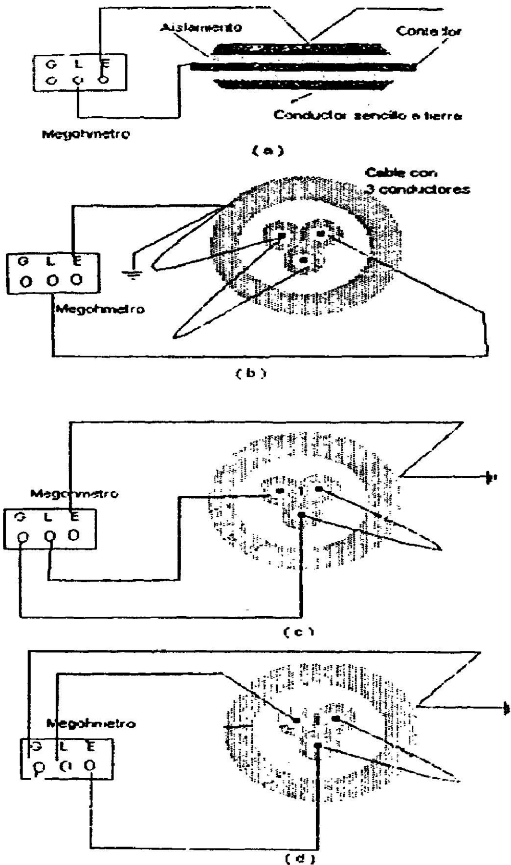
Figura 2.4 Conexiones de la prueba de cable para medición de la resistencia de aislamiento: (a) Conexión para la prueba de un conductor sencillo y un conductor a tierra. (b) Conexión para un cable de tres conductores, un conductor a otro conductor y el envoltente a tierra. (c) Conexión para un cable de tres conductores, un conductor a la vaina y a tierra y dos conductores protegidos. (d) Conexión para un cable de tres, un conductor a todos los otros conductores sin pérdidas por tierra.
