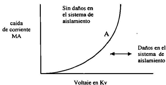
Fig. 2.5 Paso de voltaje alto - potencial prueba de corriente.
