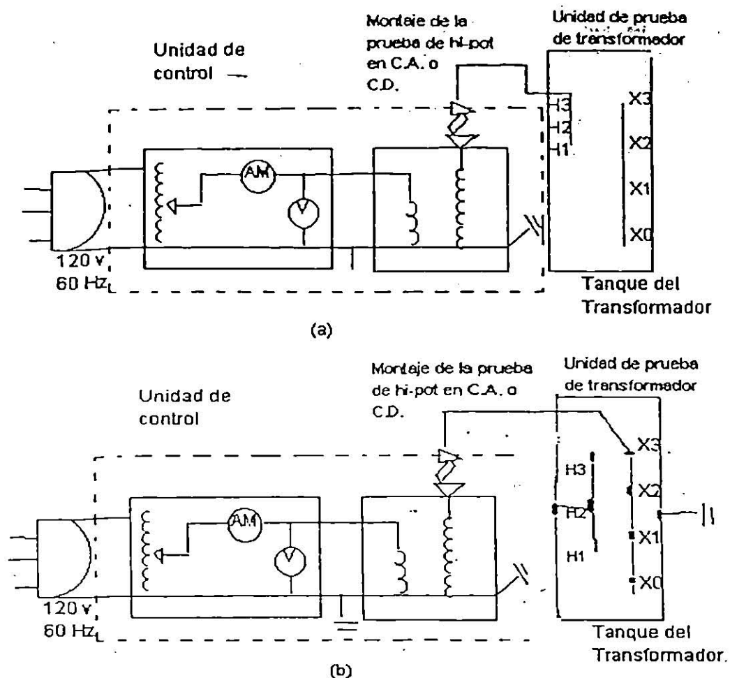
Fig. 2.3 Conexión de la prueba de alto voltaje del transformador ( HI – POT ). (a) Conexión de la prueba HI – POT en las bobinas de alta. (b) Conexión de la prueba HI – POT en las bobinas de baja.
