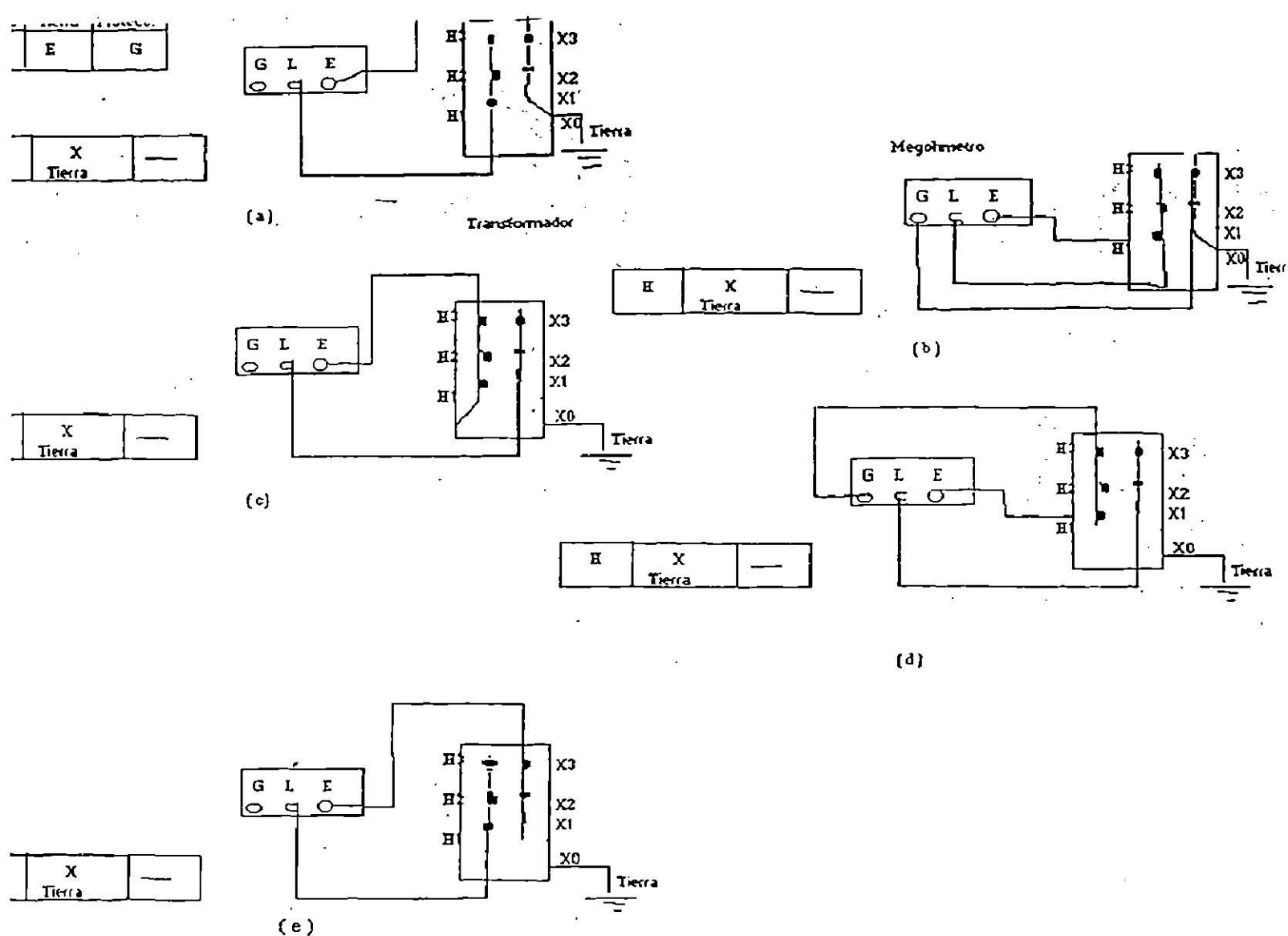
Fig. 2.2 Conexiones de prueba para resistencia de aislamiento para transformadores trifasicos. ( a ) Conexiones de bobina de alta a bobina de baja a tierra; ( b ) Conexión para bobina de alta a tierra y bobina de alta protegida; ( c ) Conexión de bobina de baja a bobina de alta a tierra; ( d ) Conexión de bobina de bobina de baja a tierra y bobina de alta y protegida; ( e ) Conexión de bobina de alta a bobina de baja.
