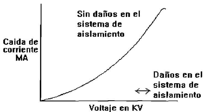
Figura 2.6 Paso de voltaje alto - potencial prueba de corriente.
