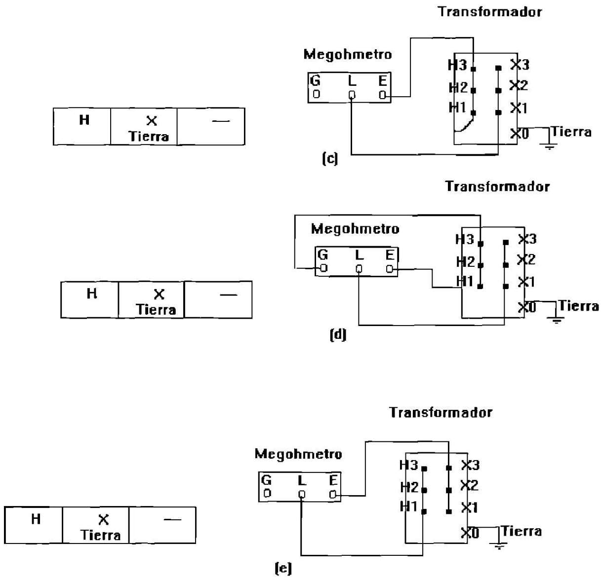
FIG. 2.2 Conexiones de Prueba para resistencia de aislamiento para transformadores trifásicos. (a) Conexión de bobina de alta a bobina de baja a tierra; (b) Conexión para bobina de alta a tierra y bobina de alta protegida; (c) Conexión de bobina de baja a bobina de alta a tierra; (d) Conexión de bobina de baja a tierra y bobina de alta y protegida; (e) Conexión de bobina de alta a bobina de baja.
