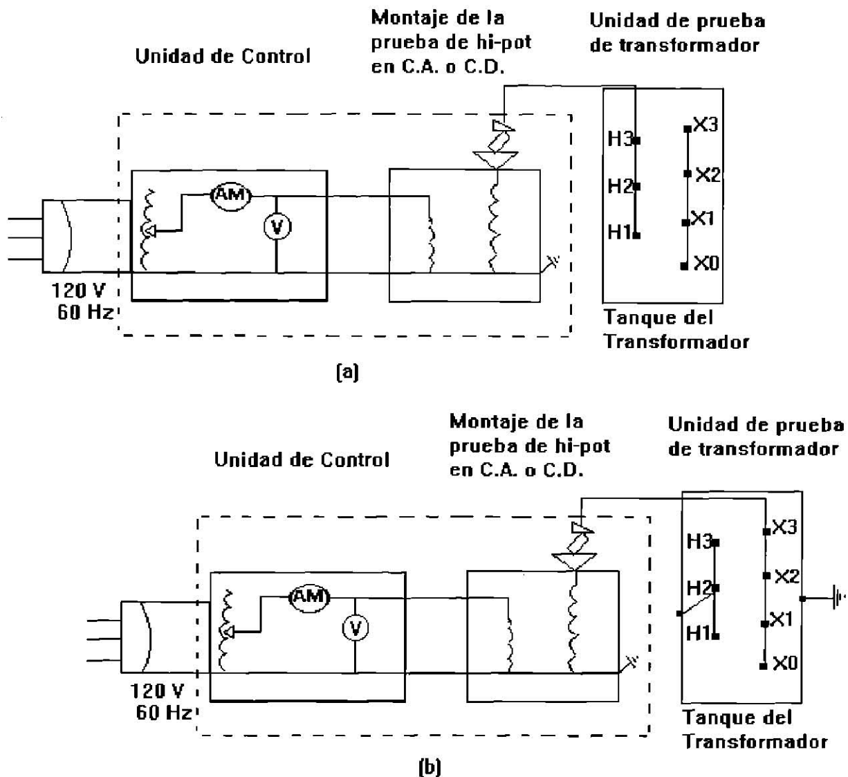
Figura 2.3 Conexión de la prueba de alto voltaje del transformador (hi-pot) a: Conexión de la prueba hi-pot en las bobinas de alta. (b) Conexión de la prueba de hi-pot en las bobinas de baja.
