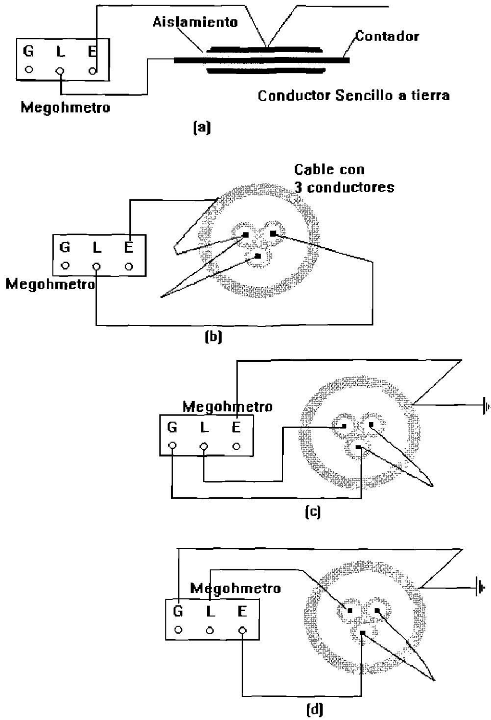
Figura 2.4 Conexiones de la prueba de cable para medición de la resistencia de aislamiento: (a) Conexión para la prueba de un conductor sencillo y un conductor a tierra. (b) Conexión para un cable de tres conductores, un conductor a otro conductor y el envoltente a tierra. (c) Conexión para un cable de tres conductores, un conductor a la vaina y a tierra y dos conductores protegidos. (d) Conexión para un cable de tres, un conductor a todos los otros conductores sin pérdidas por tierra
