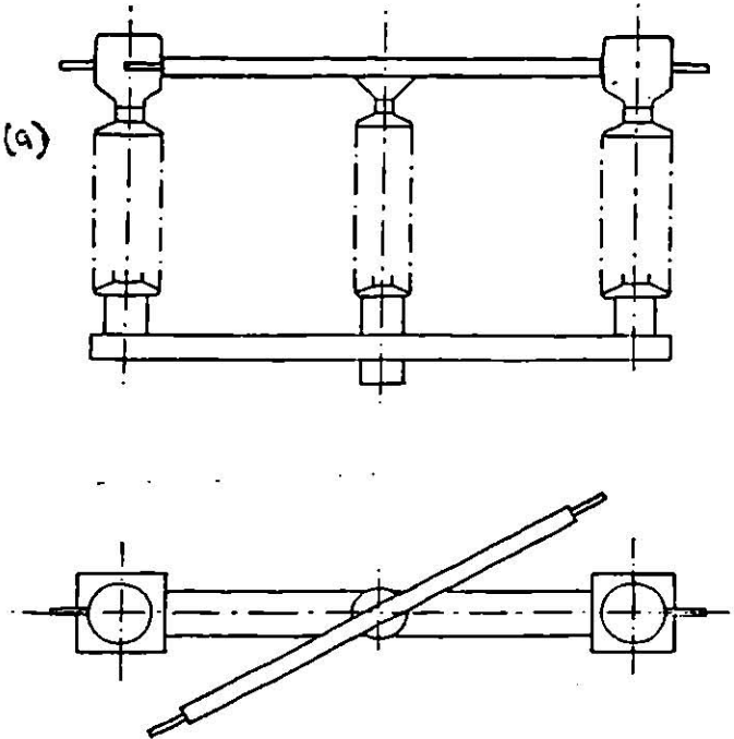
CUCHILLA DESCONECTADORA DE TRES COLUMNAS CON ACCIONAMIENTO EN LA COLUMNA CENTRAL.
