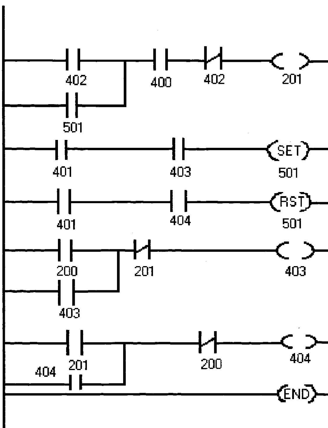
DIAGRAMA ESCALERA DE UN CONTROL DE UN NIVEL EN UN TANQUE
