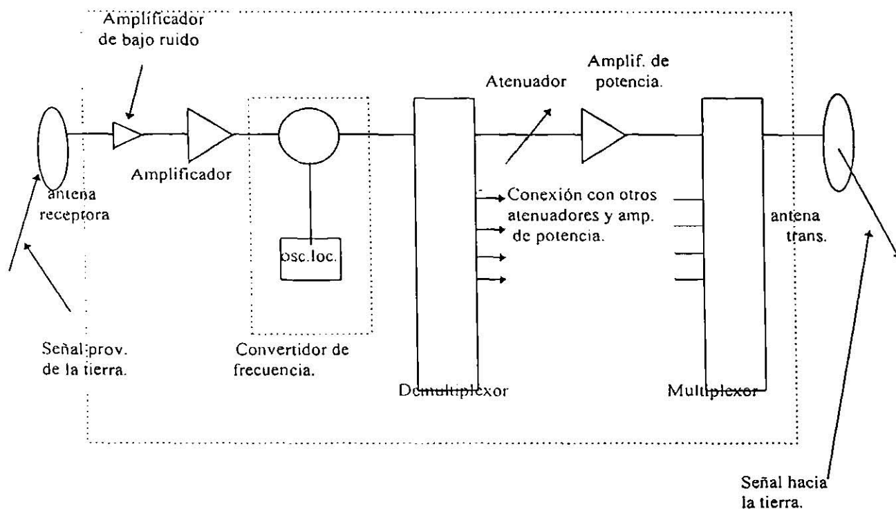
Fig. 3.7 Relación entre los subsistemas de antenas y comunicaciones.
