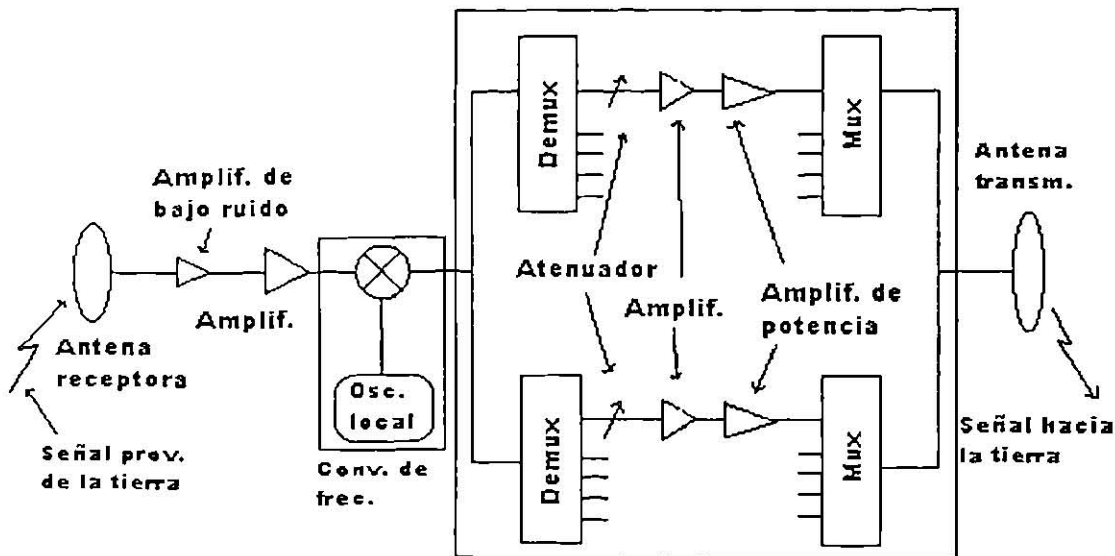
Fig 3.13 Versión modificada del diagrama y equipos del sistema de comunicaciones. A dif. del de la fig. 3.7 , se utilizan dos demultiplexores y dos mux para procesar por separado los canales pares e impares y reducir la interferencia.
