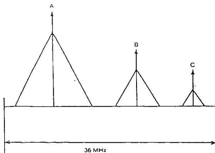
Figura 3.14 Ocupación de un transpondedor de 36 MHz con acceso múltiple por división en frecuencia; cada señal proviene de una población diferente y tiene su propia frecuencia portadora asignada.
