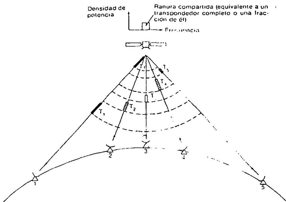
Figura 3.21 Red de cinco estaciones terrenas que comparten una misma ranura de frecuencia en un transpondedor mediante acceso múltiple por división en el tiempo con asignación fija y tiempos T desiguales por estación. Todas las estaciones transmiten su ráfaga digital a la misma frecuencia en forma secuencial.
