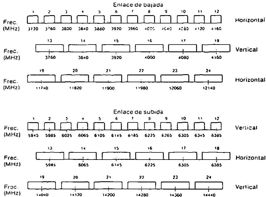
Figura 3.14 Plan de frecuencias y polarización de un satélite Spacenet. (Cortesía de GTE Spacenet Corporation.)
