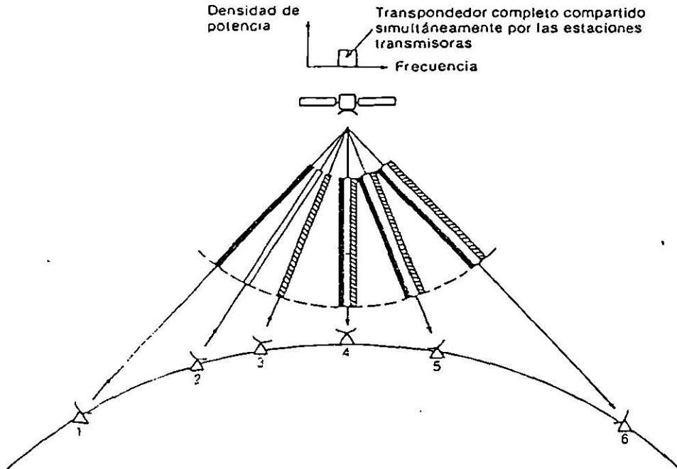
Figura 3.23 Red de seis estaciones terrenas que operan con acceso múltiple CDMA. Las estaciones transmisoras usan la misma frecuencia y transmiten al mismo tiempo; las receptoras deben conocer el código de transmisión para reconstruir el mensaje original.
